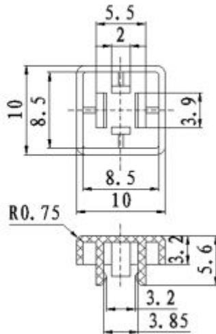
A14 Long Foot Switch Cap
